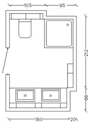
Plan prezentowanej łazienki Powierzchnia 5,5 m 2
